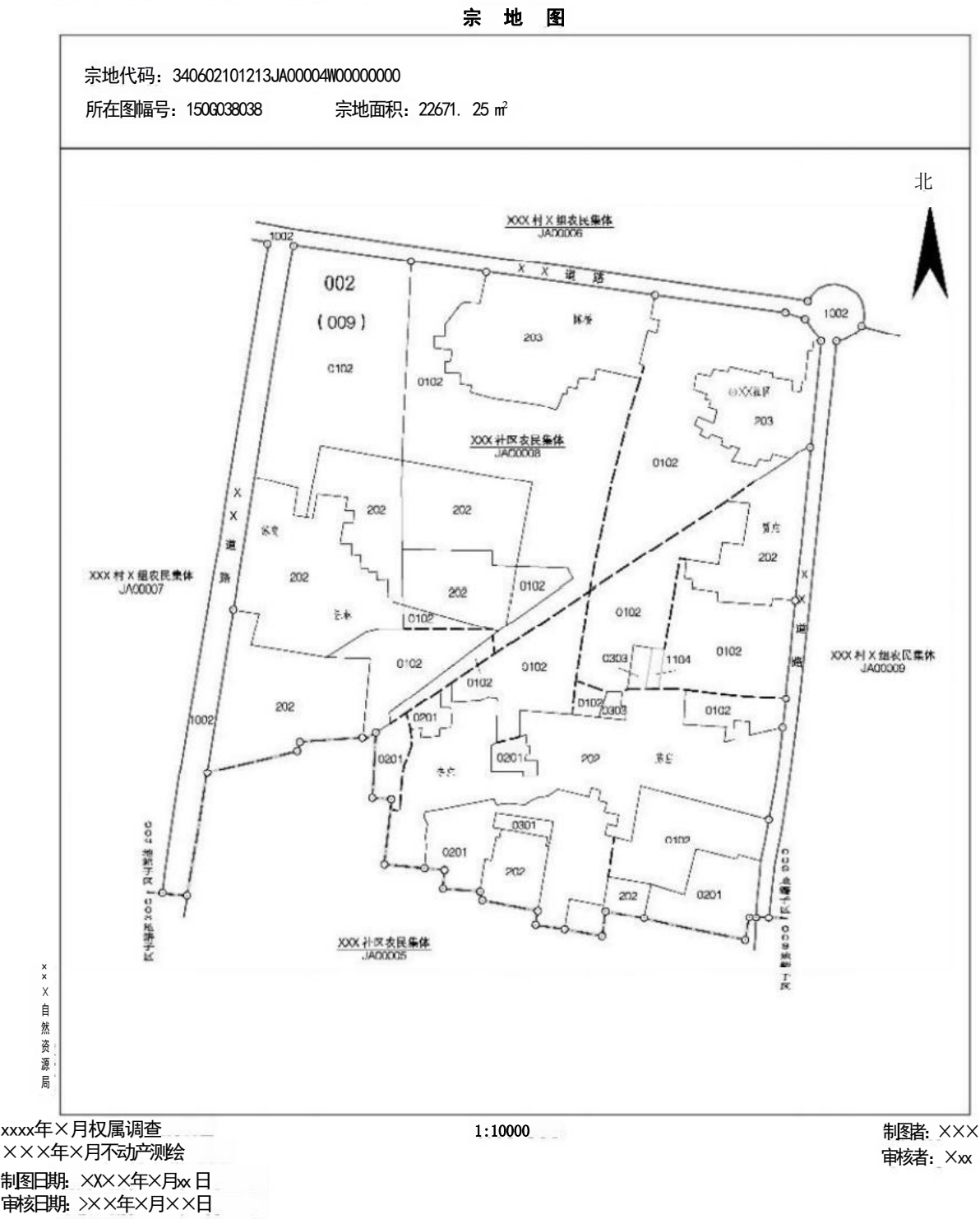
图 L. 4 土地所有权宗地图样图
