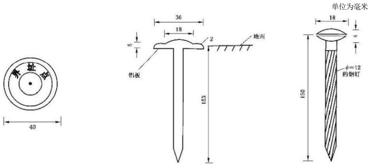
图 G.3 带铝帽的钢钉界址界标
